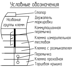
Рисунок Д.1 – Схема электрическая соединений рядов зажимов (часть 1)
